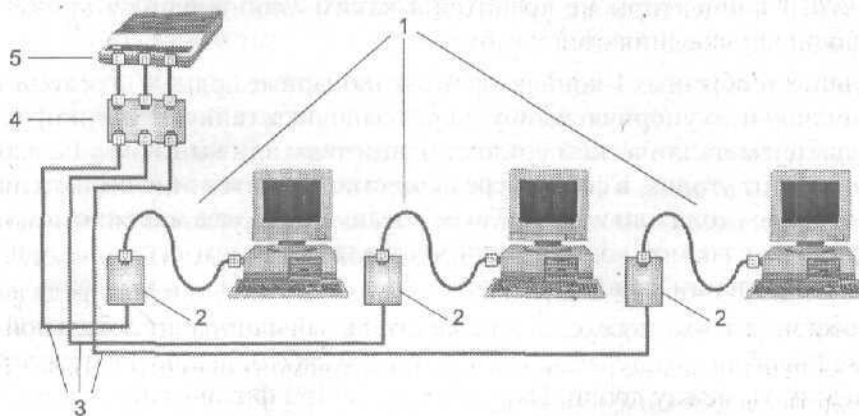
Рис. 5.8. Общая схема подключений устройств в сети IOBaseT: 1— Path Cord; 2— сетевые розетки RJ-45; 3— кабель «витая пара»; 4— path panel; 5— концентратор
