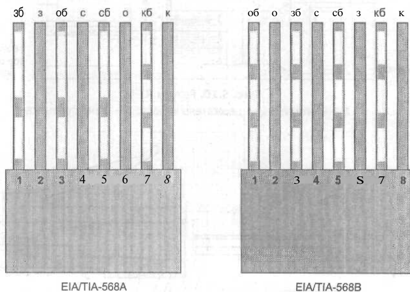
Рис. 5.12. Схемы заделки восьмижильного кабеля «витая пара»:
